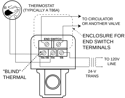
Fig. 4 - V8043F WIRING
