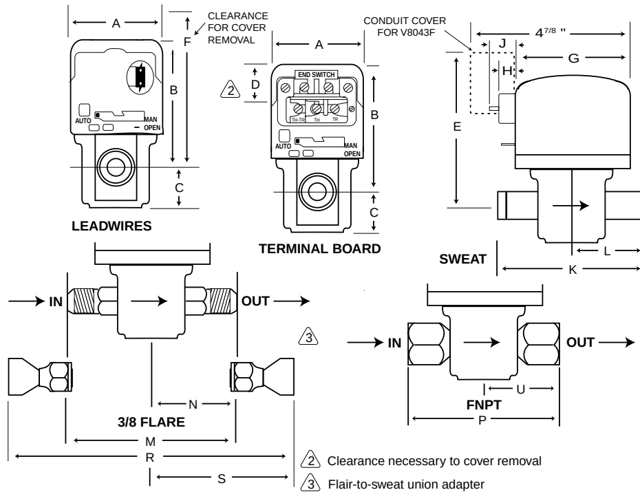
Fig. 1 - DIMENSIONS
