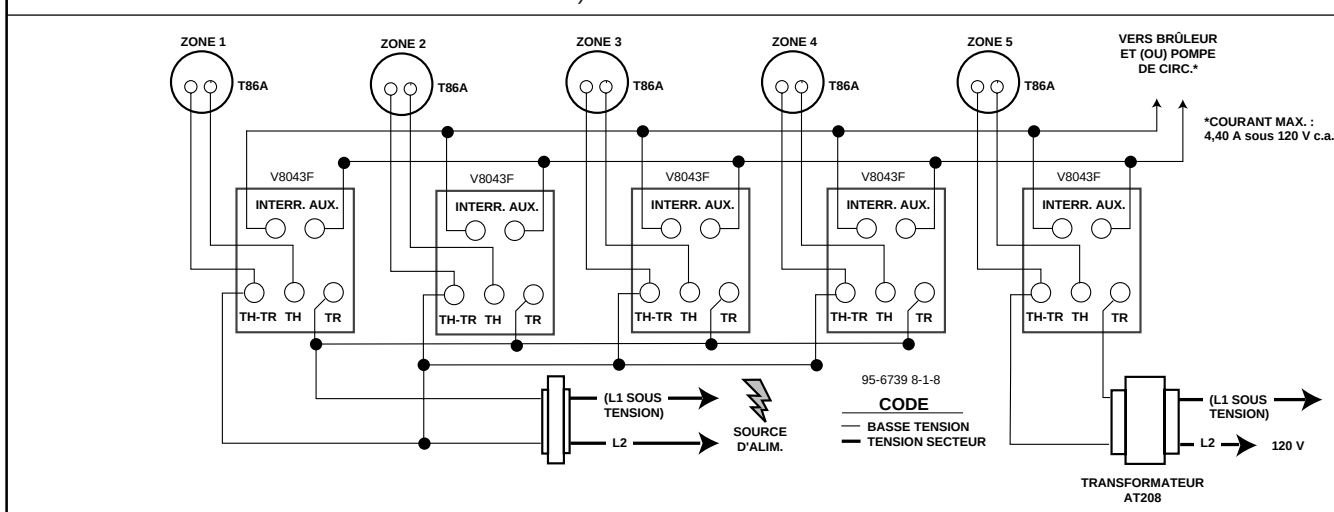
FIG. 7 - SYSTÈME À 5 ZONES AVEC TRANSFORMATEUR AT72A POUVANT ALIMENTER 4 VANNES DE ZONES (UN AT20B PEUT ALIMENTER SEULEMENT 2 VANNES)
