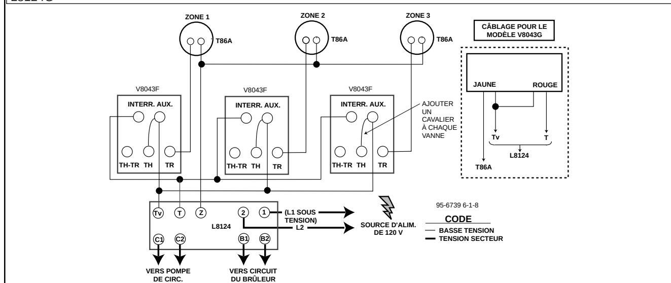
FIG. 6 - SYSTÈME À 3 ZONES AVEC TRANSFORMATEUR POUR VANNE INCORPORÉ ET RELAIS AQUASTAT L8124G
